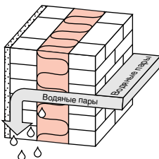
Пароизоляция
